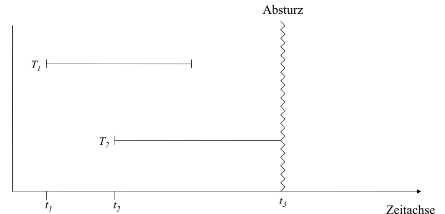
Abb.: Transaktionsbeginn und -ende relativ zu einem Systemabsturz
