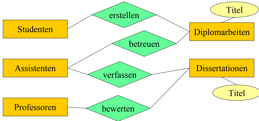
Sicht 1: Erstellung von Dokumenten als Prüfungsleistung
