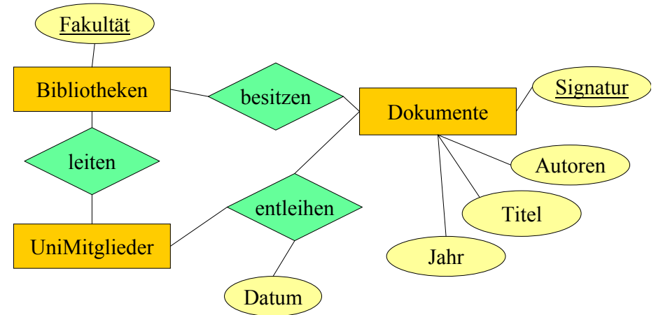
Sicht 2: Bibliotheksverwaltung
